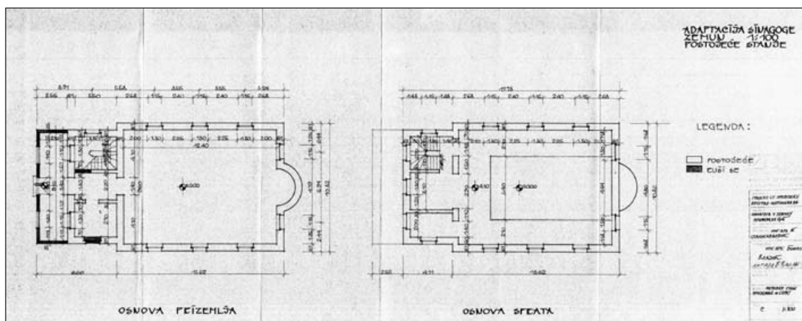
60. Postojeće stanje prizemlja i sprata pre rekonstrukcije
