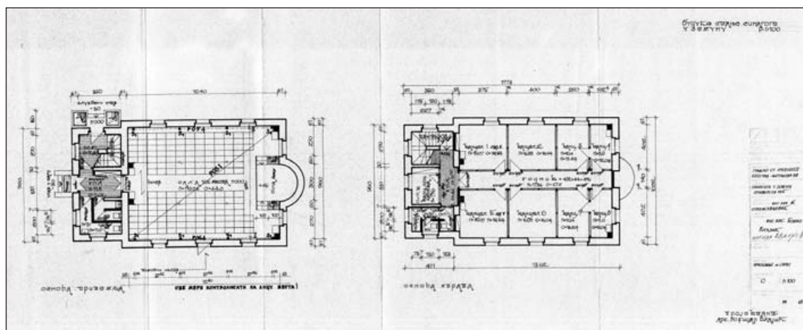
61. Plan rekonstrukcije prizemlja, sprata i izgleda fasade
